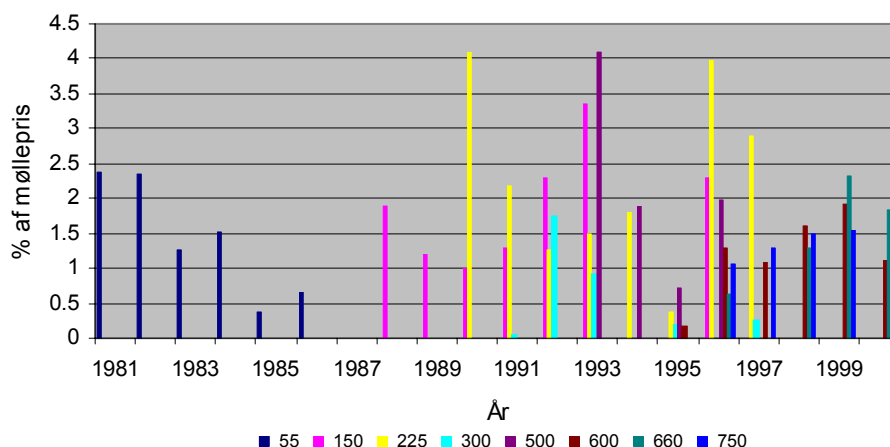
Figur 37 Vejtableringens andel i procent af mølleprisen.
