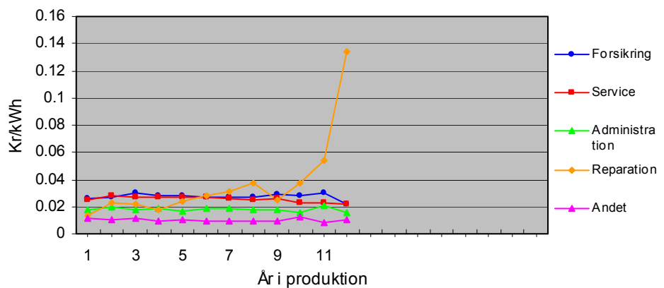
Figur 52 Udvalgte D&V poster pr. produceret kW-time for 150 kW møller (1999 – priser).
