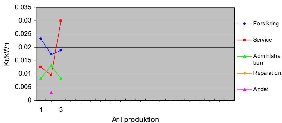
Figur 58 Udvalgte D&V poster pr. produceret kWh for 750 kW møller (1999 – priser).
