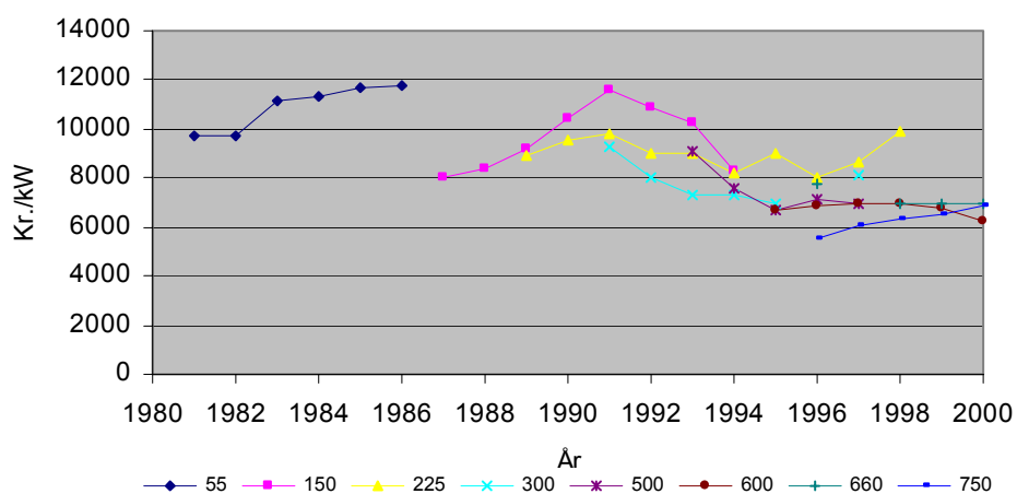
Figur 11 Samlede omkostninger som funktion af tid og installeret effekt.
