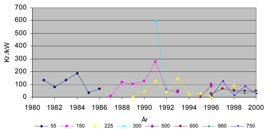
Figur 39 Andre omkostninger som funktion af tid og installeret effekt.
