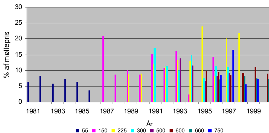
Figur 25 Netttilslutningens andel i procent i forhold til mølleprisen.
