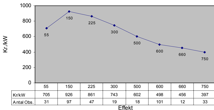
Figur 23 Netttilslutningens prisudvikling i forhold til den installerede effekt.
