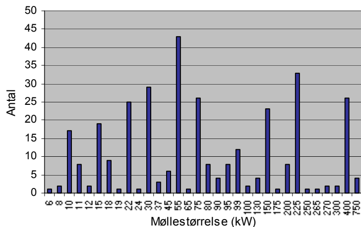
Figur 68 332 registrerede ophørte vindmøller fordelt på effektklasser.
